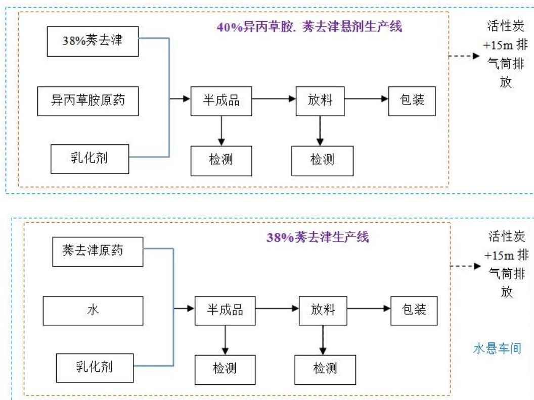
图 4.1-3 水悬车间生产工艺流程图
