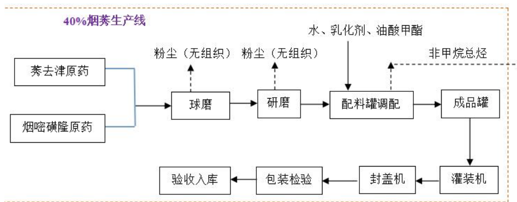
图 4.1-4 油悬车间生产工艺流程图
