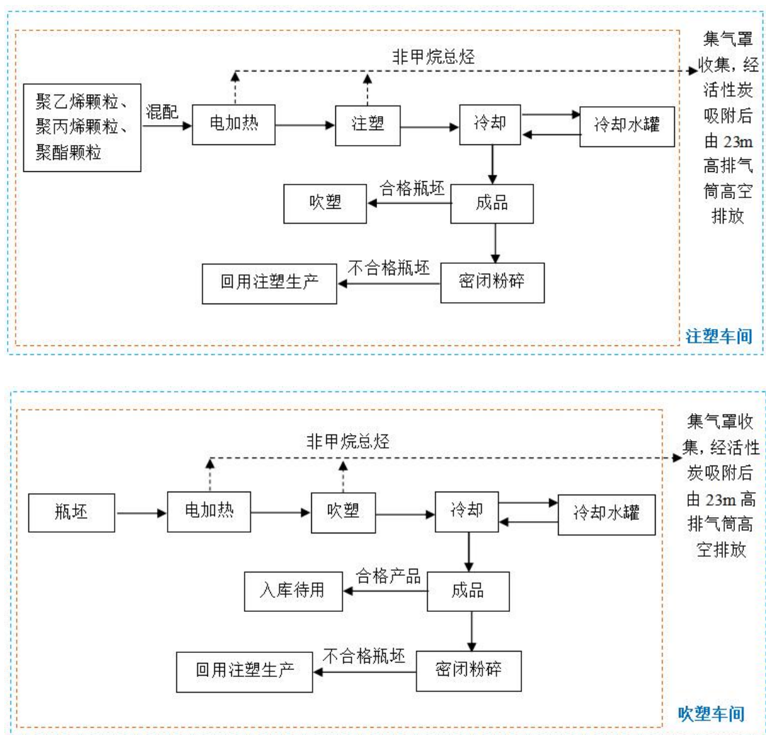
图 4.1-6 农药瓶生产工艺流程图
