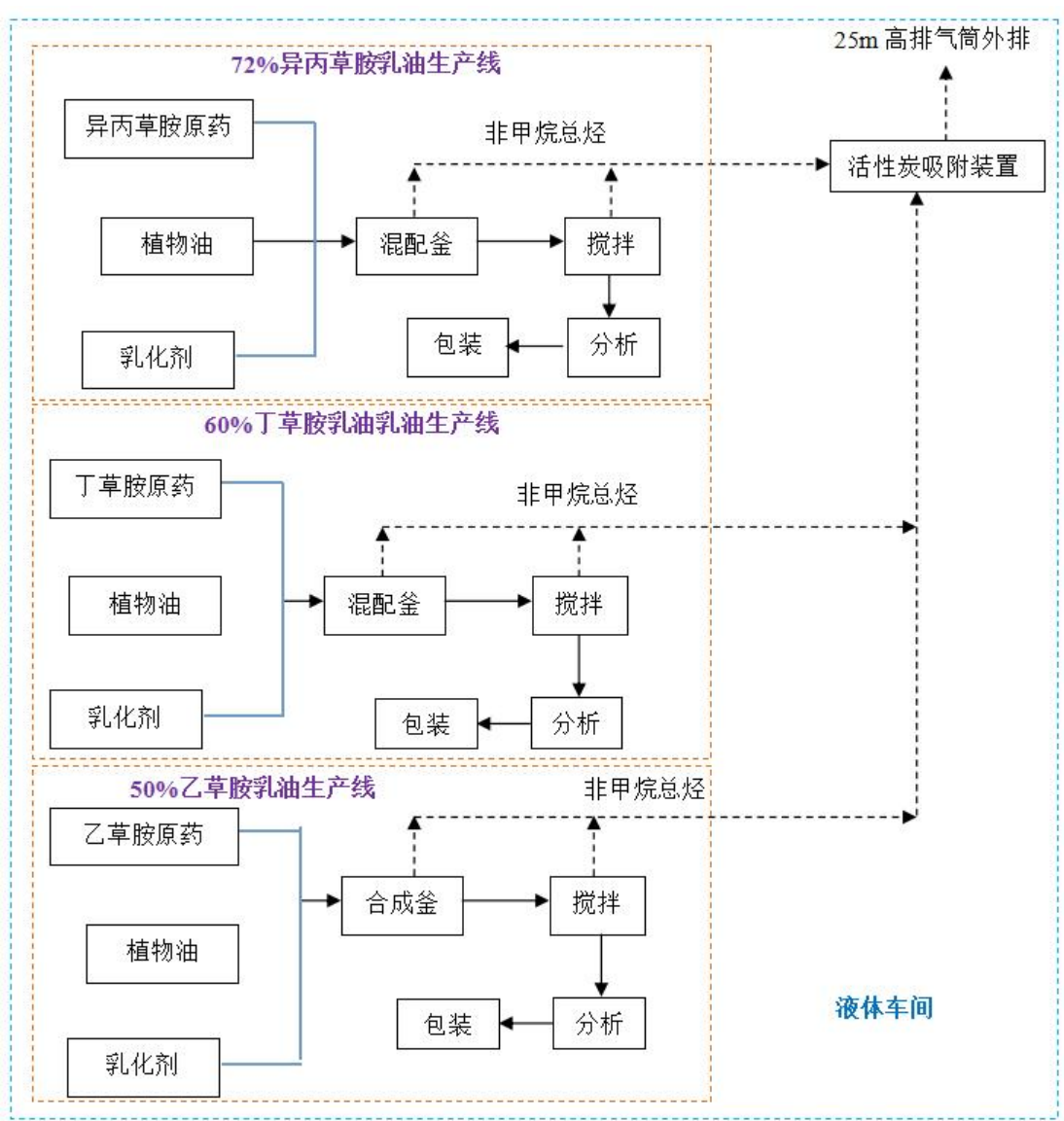
图 4.1-1 液体车间生产工艺流程图
