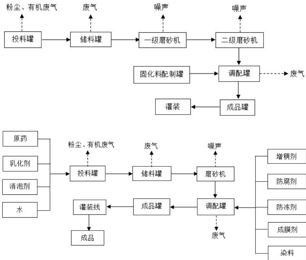
图 4.1-5 悬浮剂制剂加工车间生产工艺流程图（在建项目）
